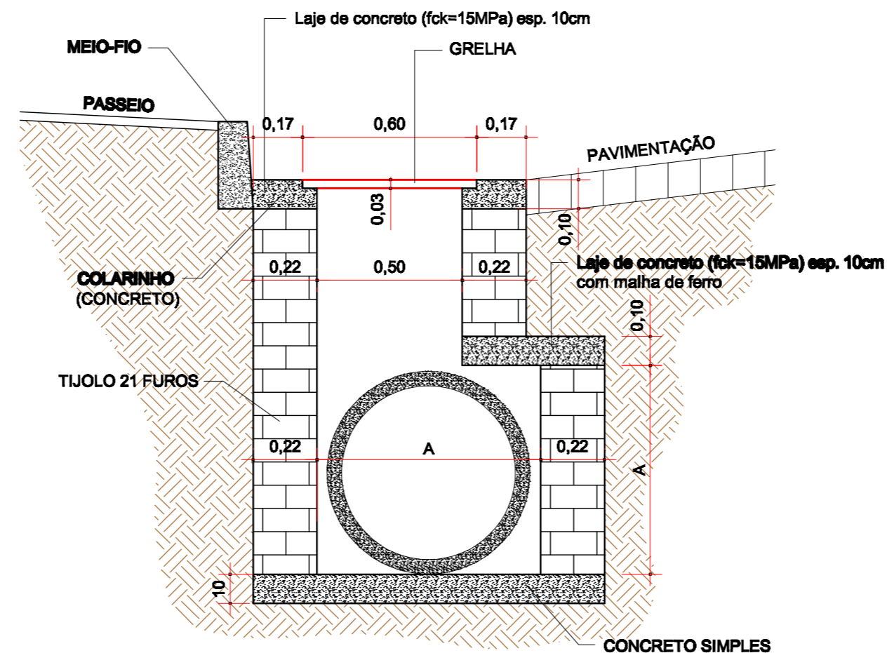
CORTE TRANSVERSAL (B B) ESC.: 1:20
