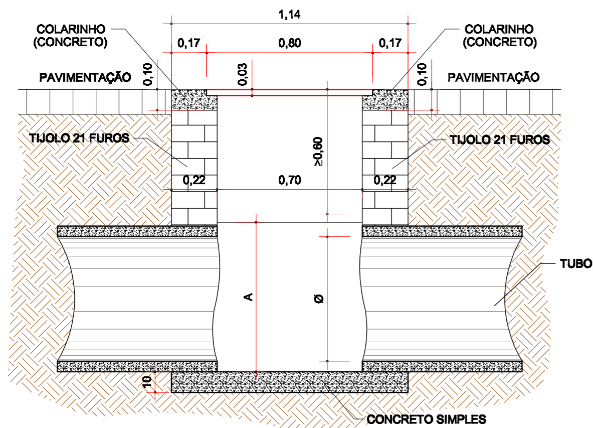
CORTE LONGITUDINAL (A A) ESC.: 1:20
