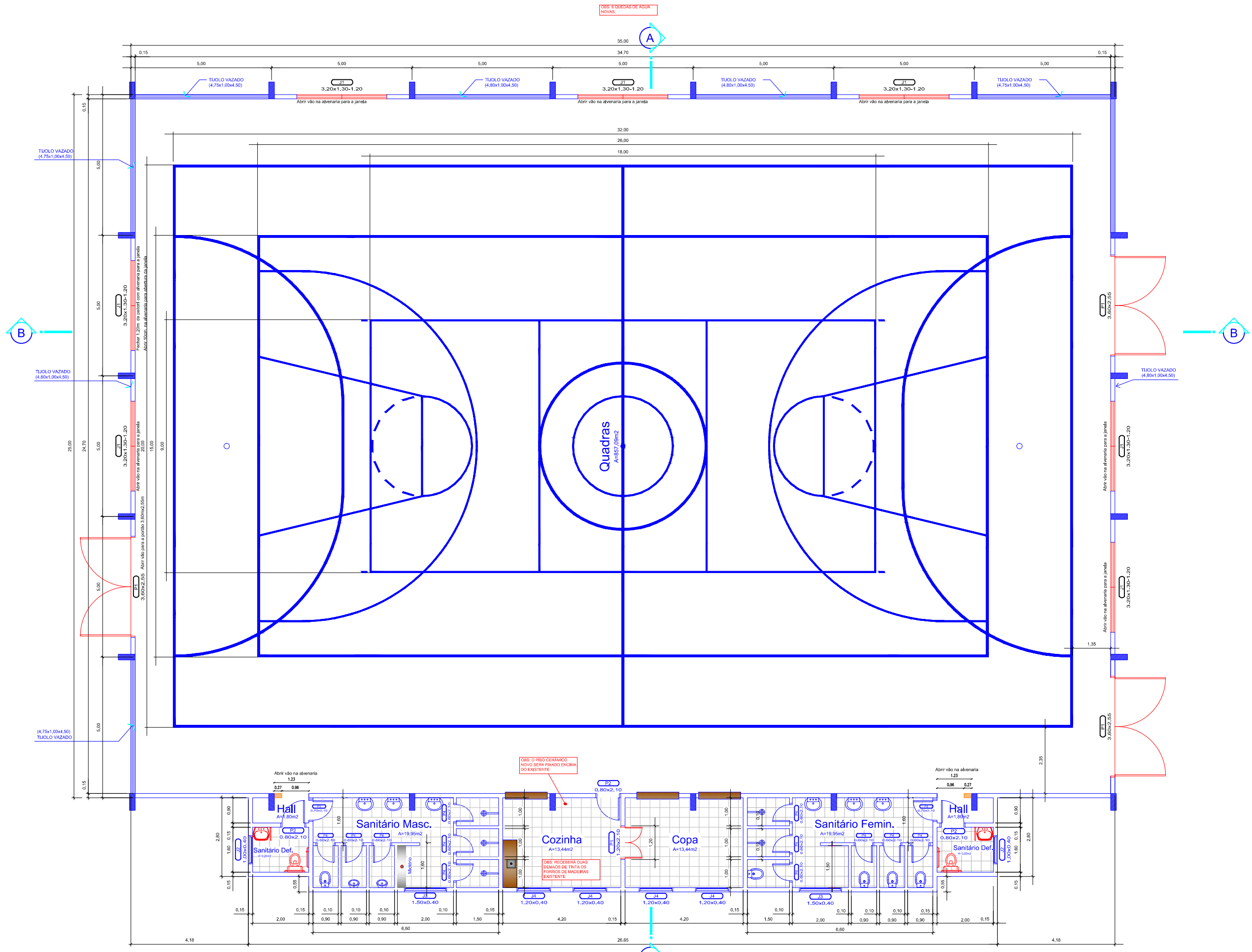
PLANTA BAIXA ESC: 1:75 ÁREA=961,91m2
